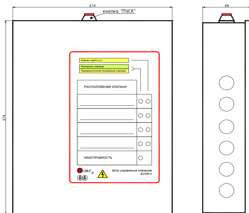
Рис 1.1 Внешний вид и габаритные размеры БУОК-4 для управления клапанами с электромеханическим приводом.
